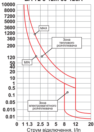
ВА-72 8-12In 80-125A
