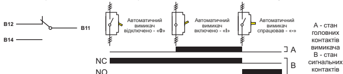
Мал. 2.7 - принципова схема та діаграма положень сигнального контакту
