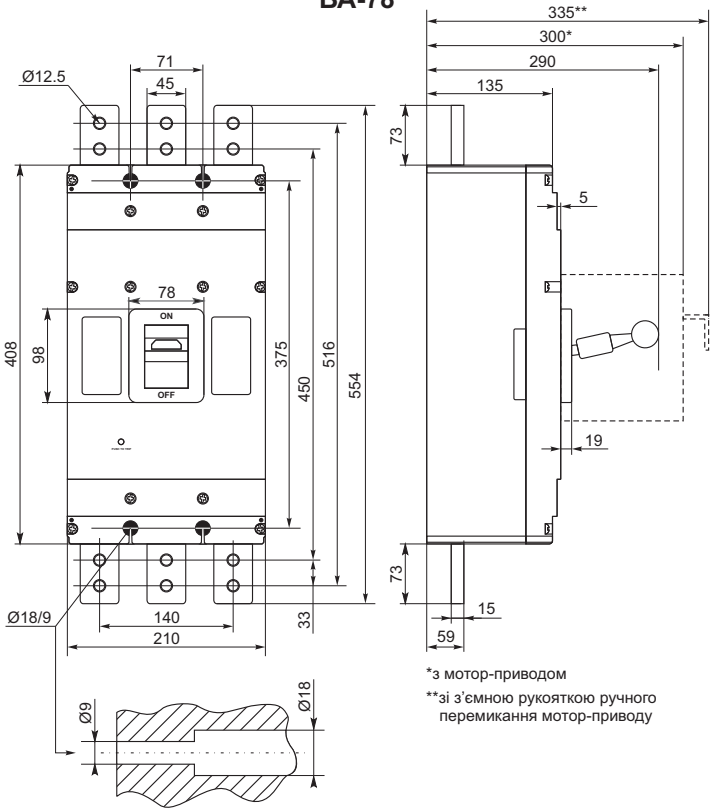
Додаток 3 - габаритні та установчі розміри автоматичних вимикачів ВА-7
