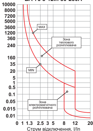
ВА-73 8-12In 80-250A
